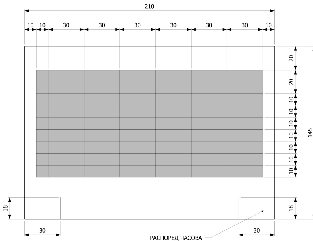
Предња страна распореда (димензије и позиција таблице)
